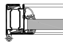
Anschweißband flächenbündig
