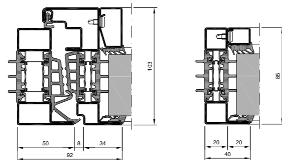
Fensterflügel-Blendenrahmen
