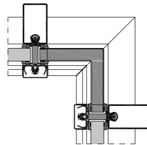
Innenecke
