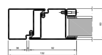
Türflügel-Blendrahmen forster presto 60s
