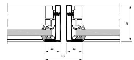
Wendetür
