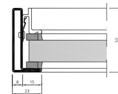
Festverglasung
