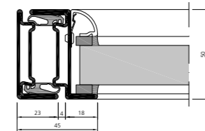
Flächenbündige Tür
