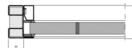
Aneinandergefügte Stossfugenverglasung
