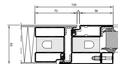
Türflügel-Blendrahmen
