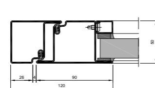
Türflügel-Blendrahmen forster presto 50
