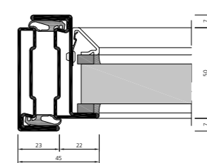
Flächenversetzte Tür
