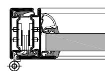
Anschraubband flächenbündig
